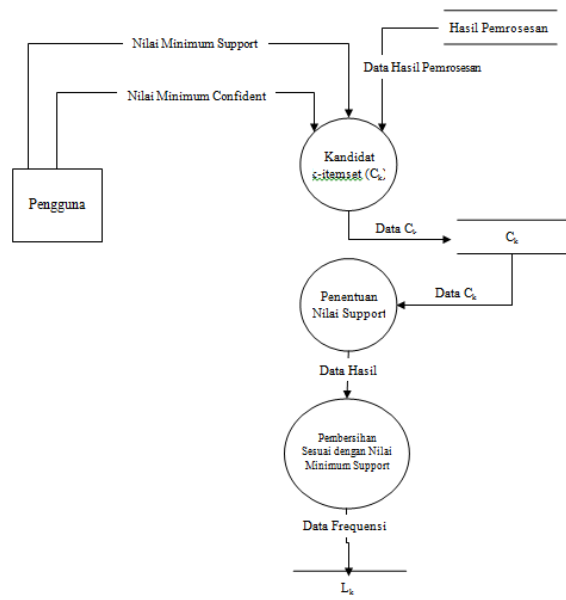
Gambar 4. DFD Level 3
