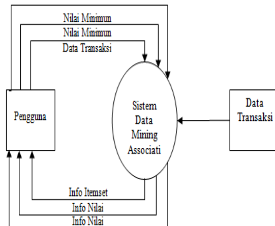
Gambar 1 Konteks Diagram
