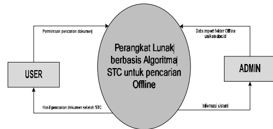
Gambar 1 Diagram Konteks
