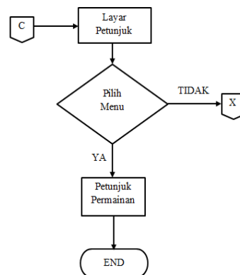
Gambar 4 Diagram Alur Petunjuk (Help)
