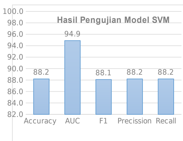
Gambar 8. Hasil Pengujian Model SVM
